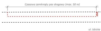
TYMCZASOWA ORGANIZACJA RUCHU – UL. IZBICKA Czasowe zajęcie pasa drogowego
